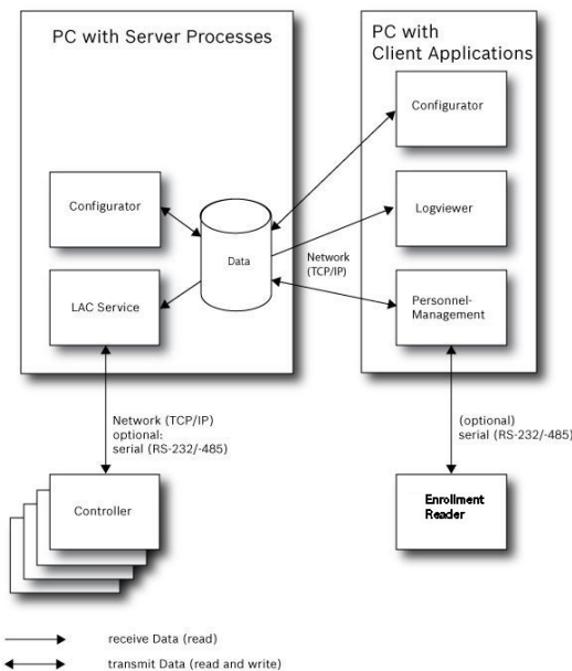
Abbildung 1.2: Systemübersicht – Verteiltes System
