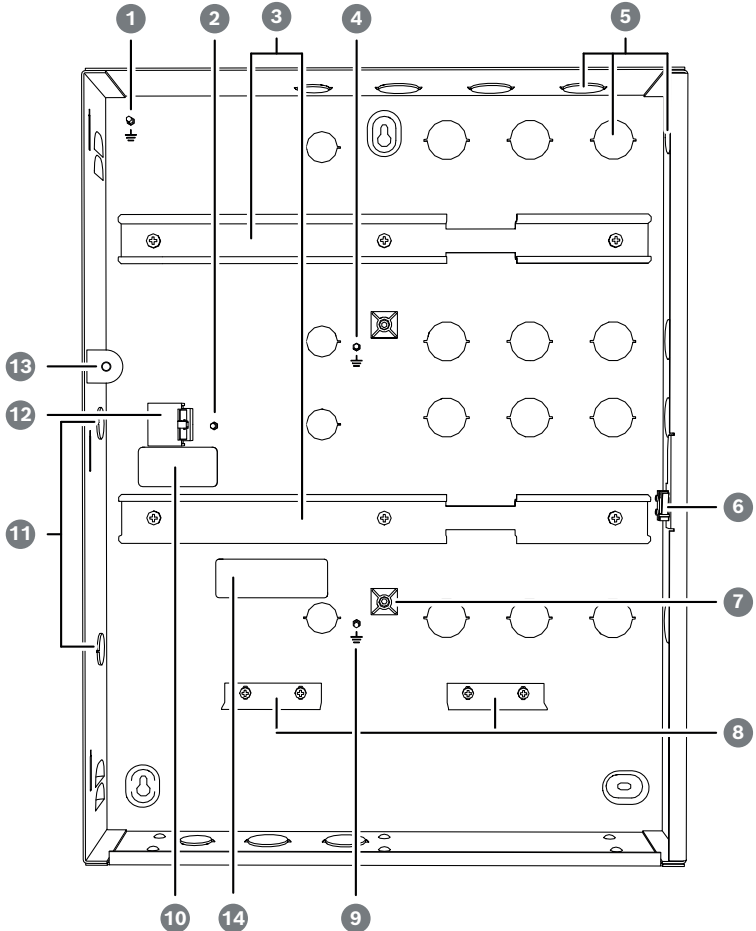
Afbeelding 1.1: Onderdelen van de behuizing
