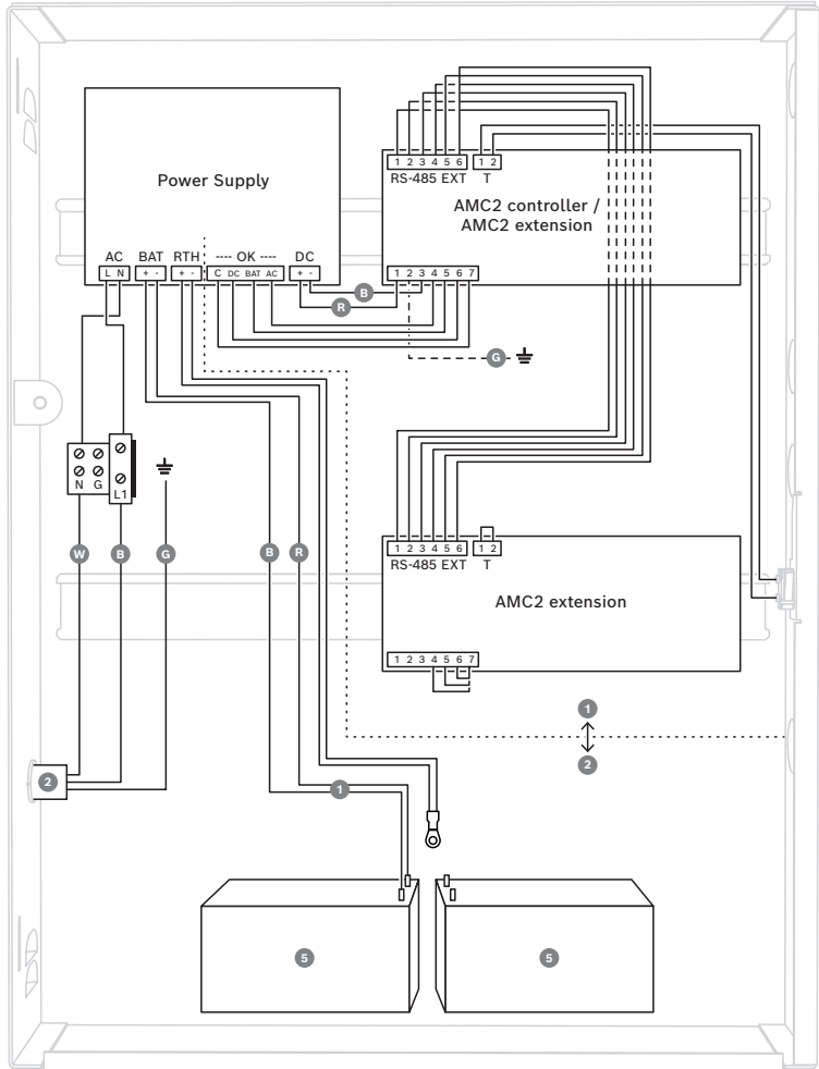
Afbeelding 3.1: Aansluitingen in de behuizing
