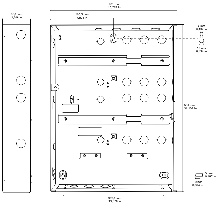
Afbeelding 2.1: Afmetingen van de behuizing
