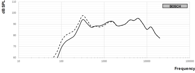
Frekans tepkisi
