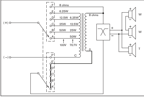
Devre şeması
