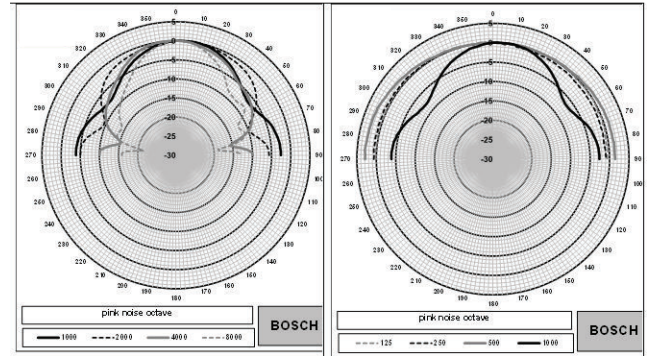
Polardiagramme
