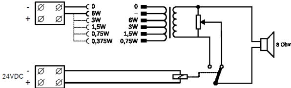
Schaltbild
