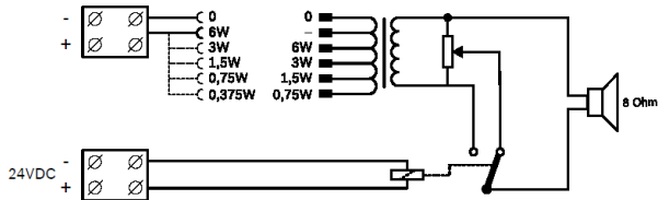
Diagrama de circuitos
