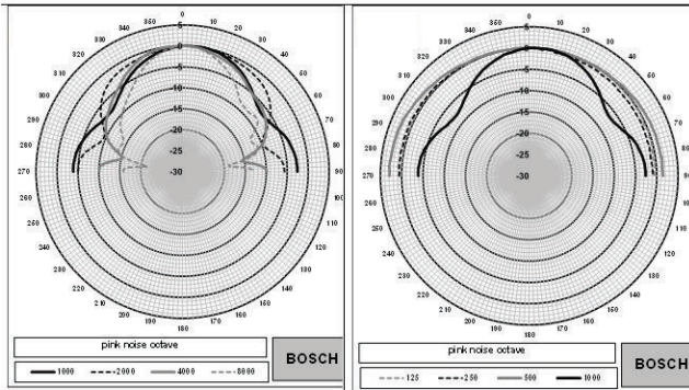
Diagramas polares
