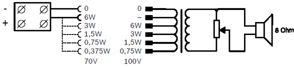
電路圖
