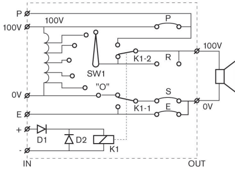
LBC 1401/10 devre şeması
