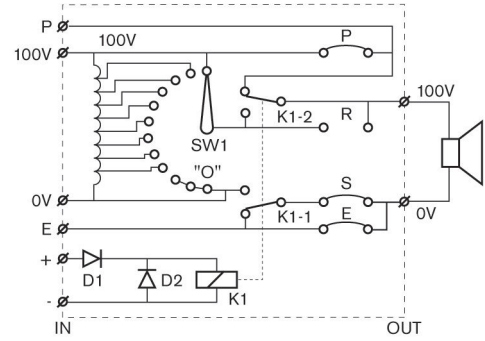
LBC 1411/20 devre şeması
