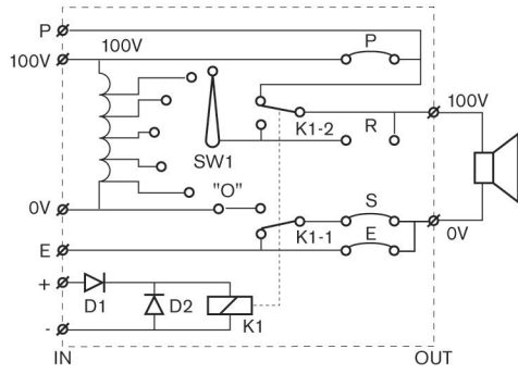
LBC 1401/20 devre şeması
