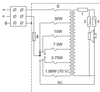
Sơ đồ nối mạch (1: Bộ giới hạn Thụ động, 2: Bộ Lọc Tần Số Thấp, 3: Bộ Lọc Tần Số Cao, 4: Cầu chì nhiệt)
