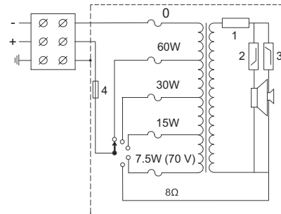
회로도(1: 수동 리미터, 2: 로우 패스 필터, 3: 하이 패스 필터, 4: 온도 퓨즈)
