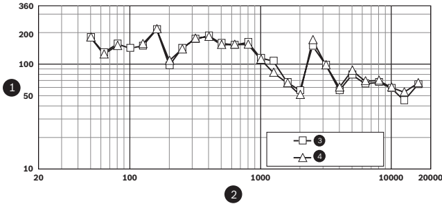
주파수 응답
