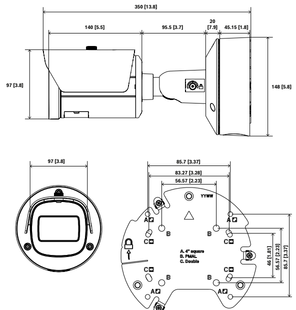
Размеры в мм (дюймах)
