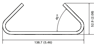
尺寸 (单位: 毫米 (英寸))
