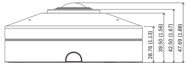
Dimensioni in mm (pollici)
