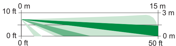
侧视图
