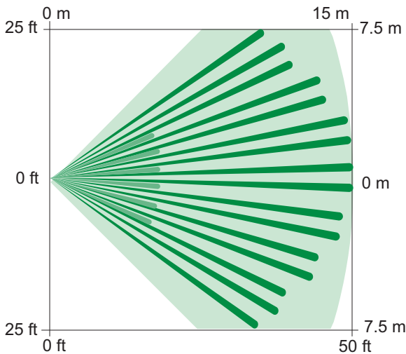
俯视图
