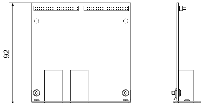
Abb. 2: Abmessungen
