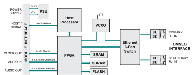
Abb. 1: Schaltbild
