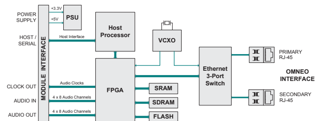
Fig. 1: Schéma du circuit
