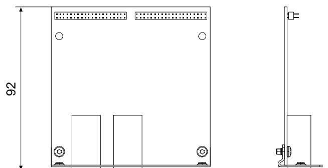
Fig. 2: Dimensions
