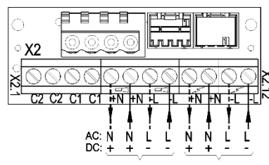
Betriebsspannungsanschluss Schallgeber
