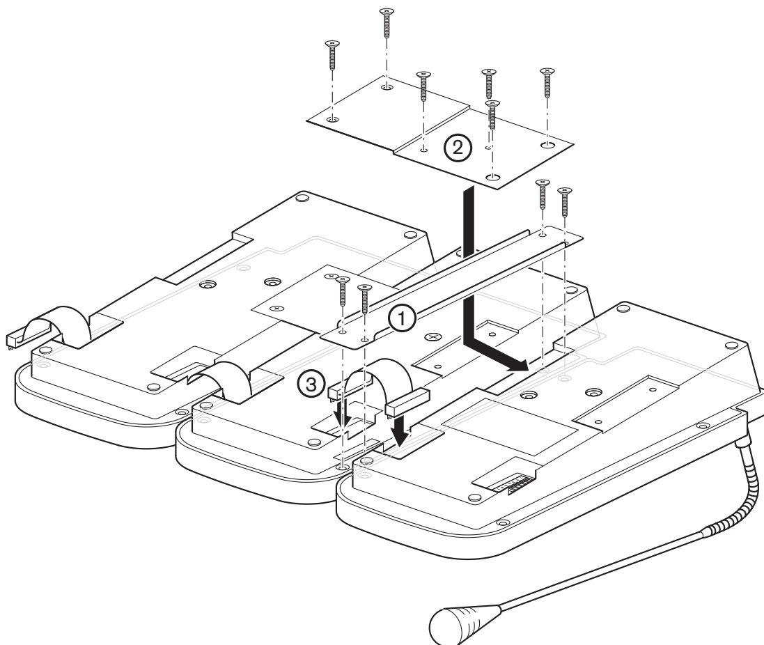
Figura 4.2: Conexión de teclados de estaciones de llamada
