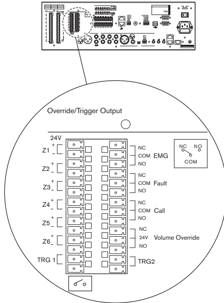
Figura 5.7: Salidas de regulación
