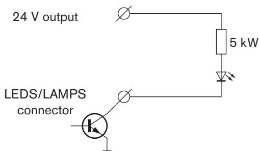
Figura 5.26: Conexión de los LED
