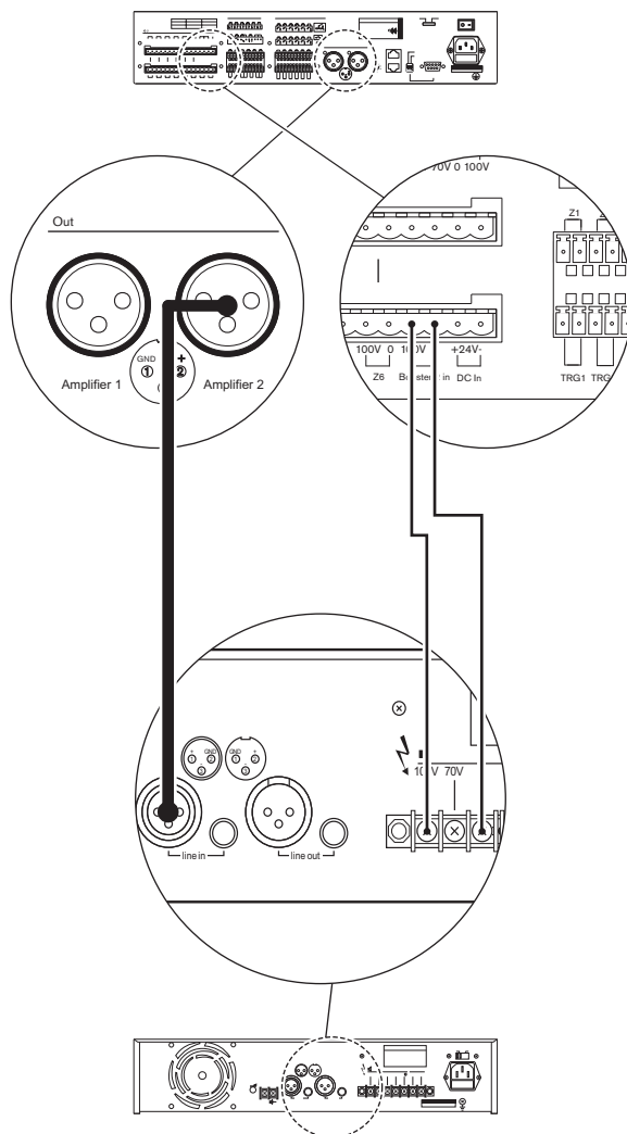
Figura 5.22: Conexión del amplificador de potencia externo 2
