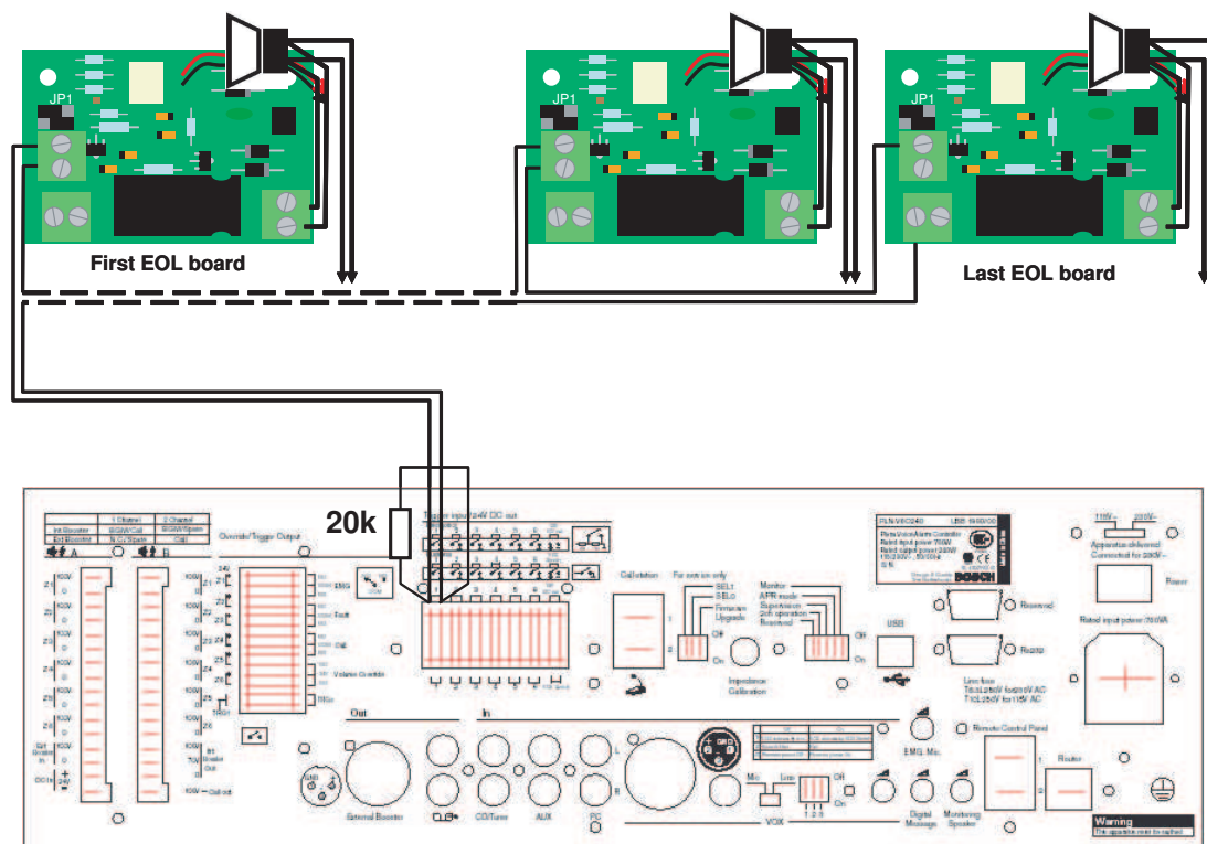
Figura 4.5: Indicación de entrada de activación
