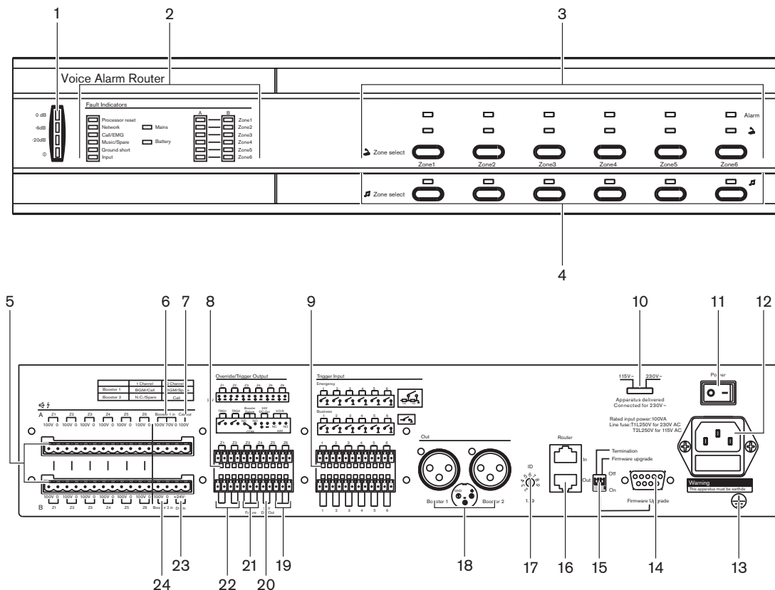
Figura 3.4: Vistas frontal y posterior del enrutador de alarma por voz Controles, indicadores y conectores del enrutador de alarma por voz:
