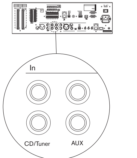
Figura 5.14: Entradas de música ambiental
