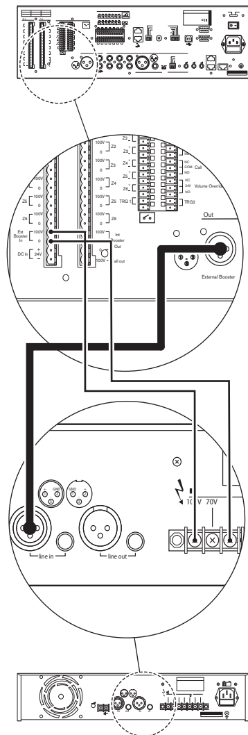
Figura 5.4: Conexión de un amplificador de potencia externo
