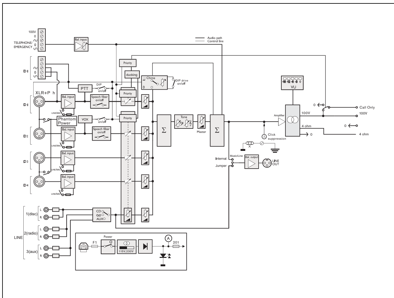
figura 2.1: Panoramica schematica del Plena Mixer Amplifier
