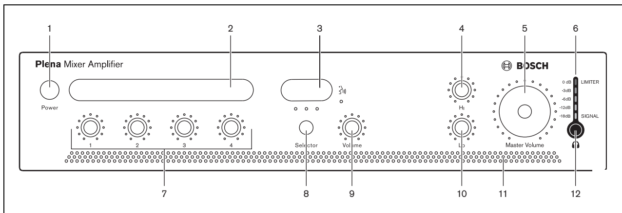
figura 2.2: Pannello frontale
