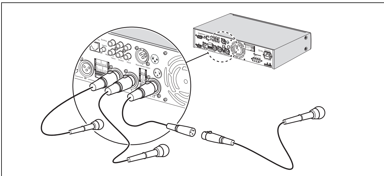
figura 4.4: Connessione degli ingressi per microfono
