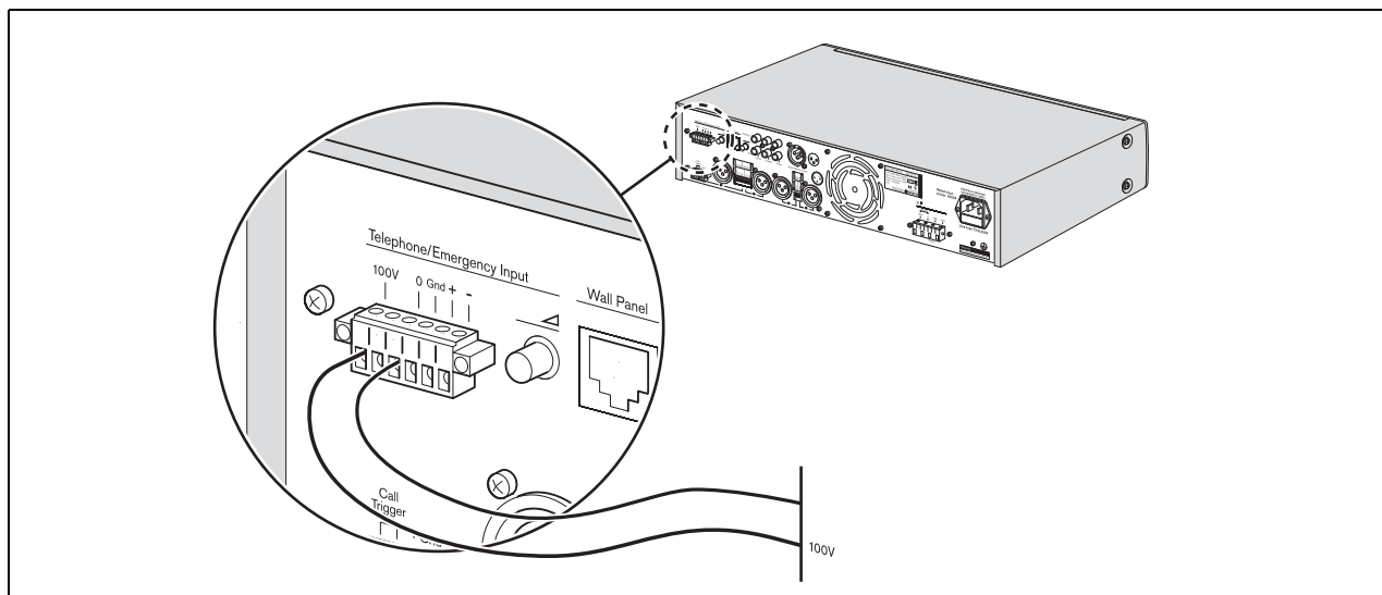
figura 4.5: Connessione del segnale d'ingresso a 100 Volt
