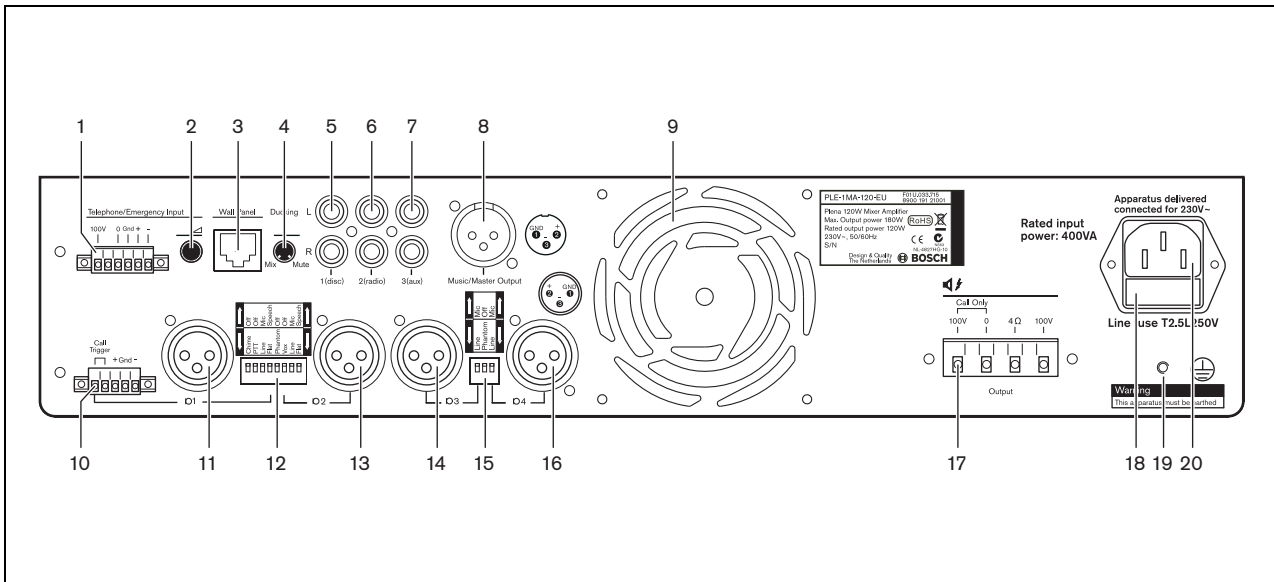
figura 2.3: Pannello posteriore
