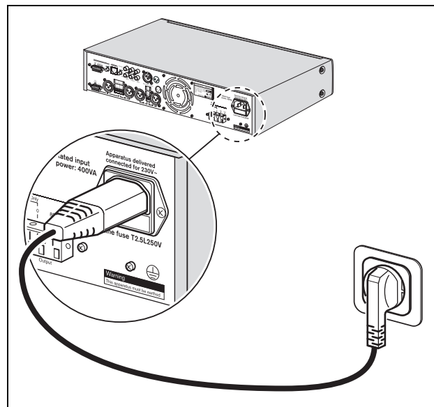
figura 3.2: Collegamento all'alimentazione e selettore di tensione
