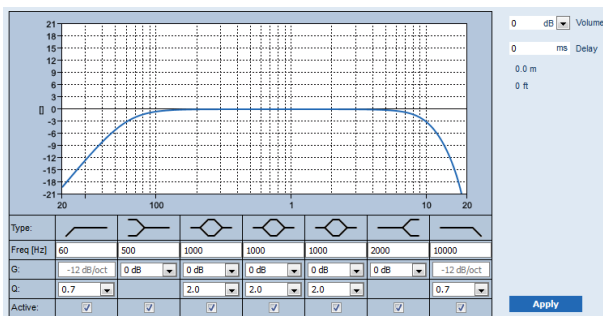
F: frekvence, G: zisk, Q: faktor kvality
