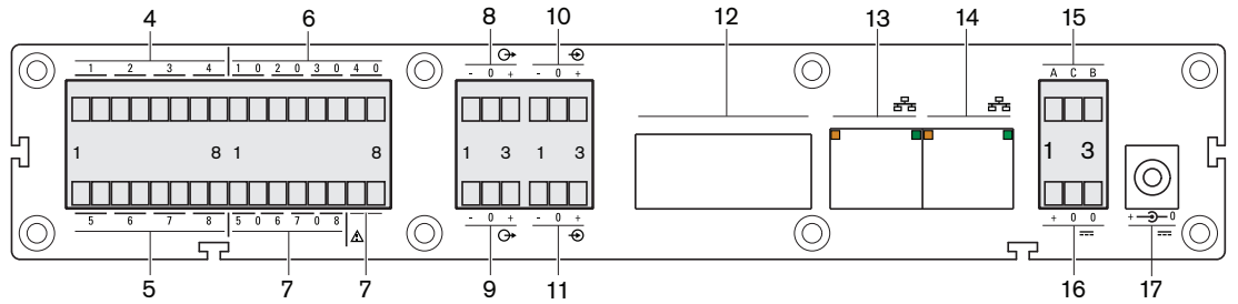
Рисунок 3.2: Вид сзади
