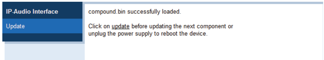
Рисунок 6.20: Подтверждение загрузки
