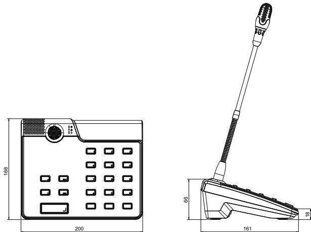
Abb. 2: Abmessungen der Sprechstelle
