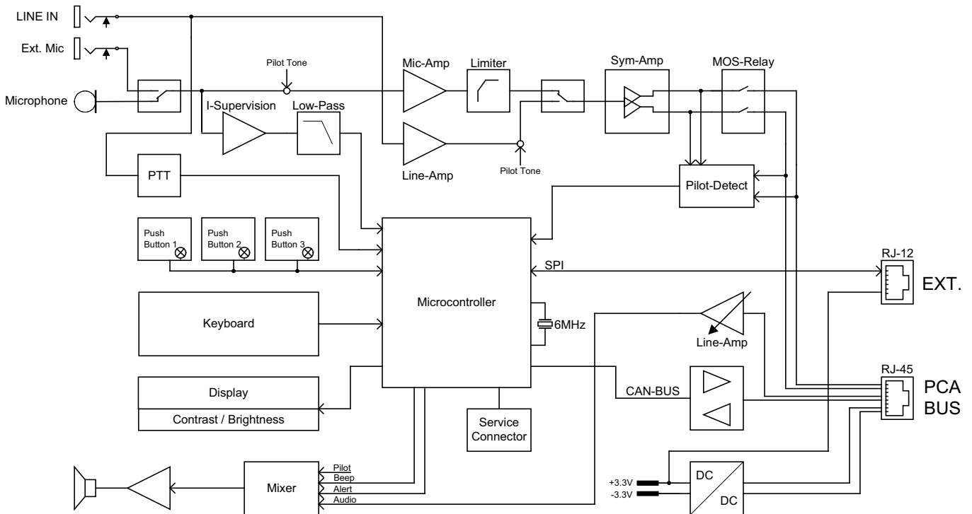
Abb. 1: Schaltbild
