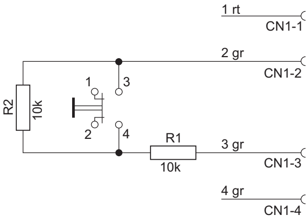
그림 2: 특수한 용도로 NOC(평소 열림 접점)로 키 스위치 연결
