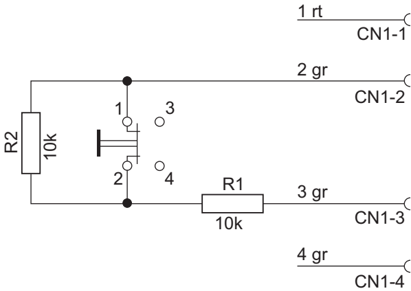
그림 1: 키 잠금 기능에 대해 NCC(평소 닫힘 접점)로 키 스위치 위치 연결
