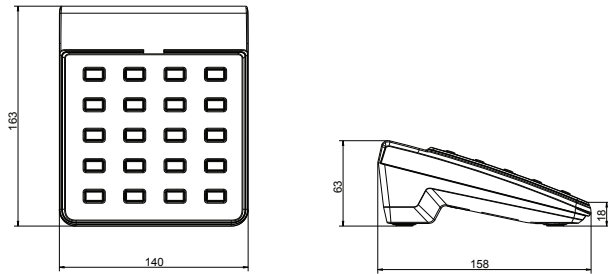
Fig. 1: Dimensions
