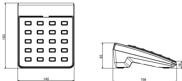
Rys. 1: Wymiary
