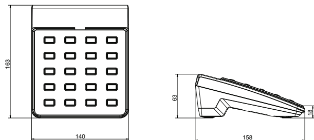
Fig. 1: Dimensões
