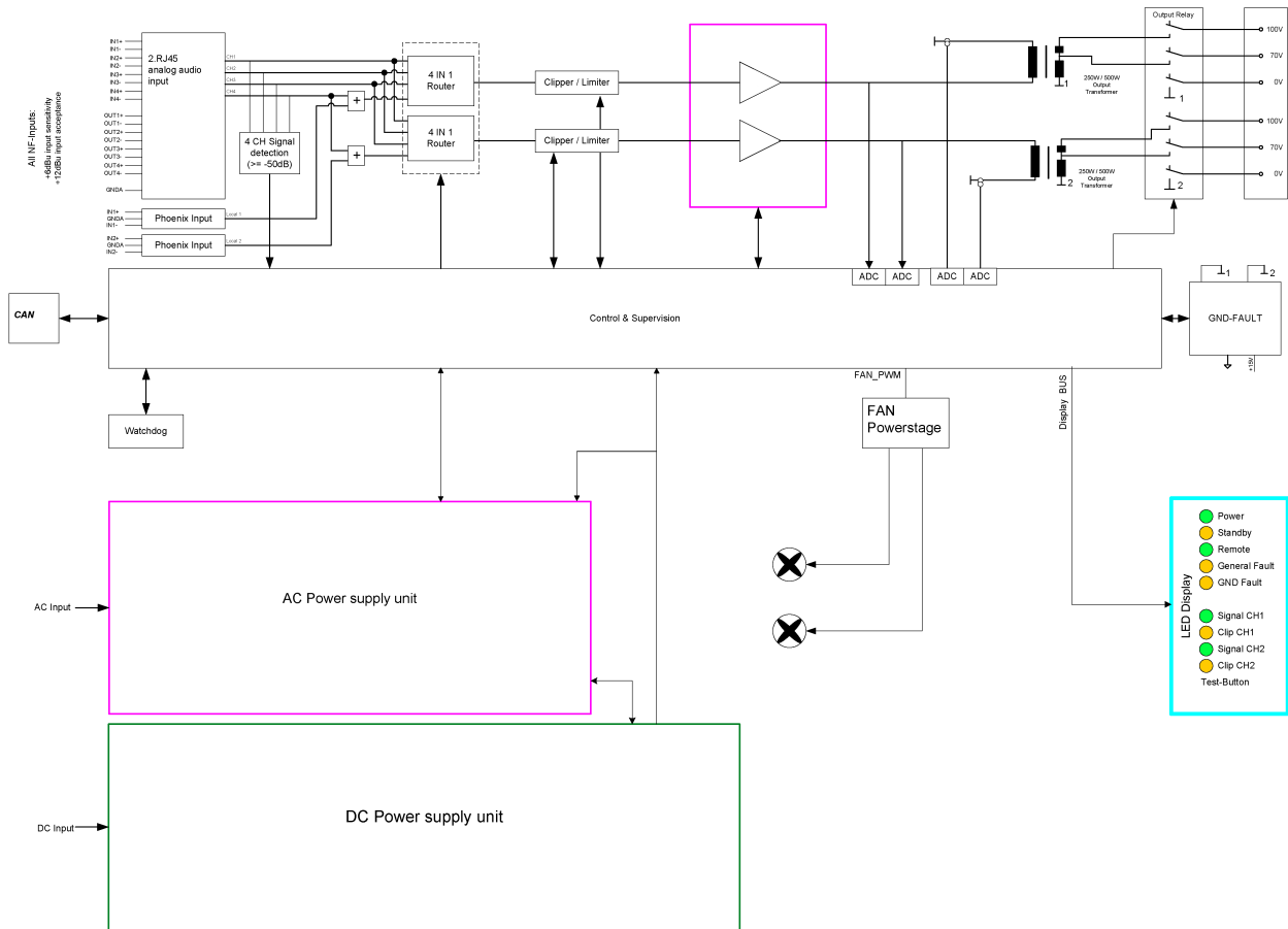
Рис. 1: Принципиальная схема
