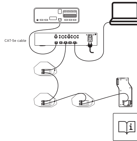
CAT-5e cable
