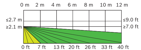
探测区域侧视图：12 米 x 12 米（40 英尺 x 40 英尺）
