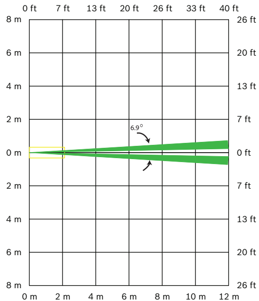
探测区域俯视图：12 米 x 1.5 米（40 英尺 x 5 英尺）
