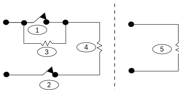
Figura 12.1: Opción de resistencia de RFL doble
