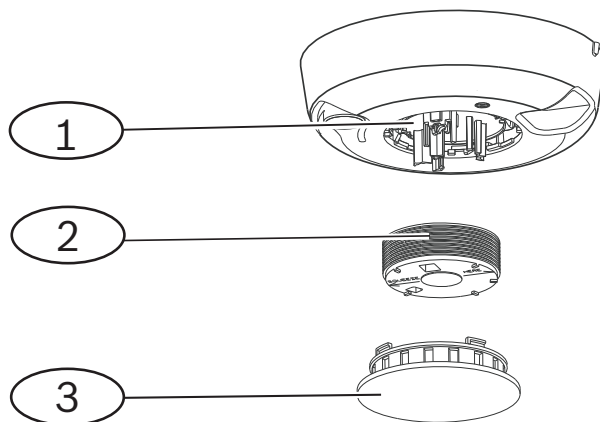
Figura 13.2: Extracción de la tapa del detector
