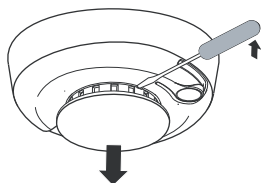
Figura 13.1: Extracción de la tapa del detector
