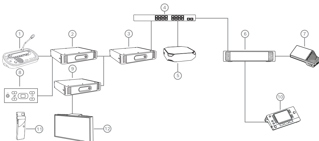
Figura 5.8: Interconectar DICENTIS con DCN NG
