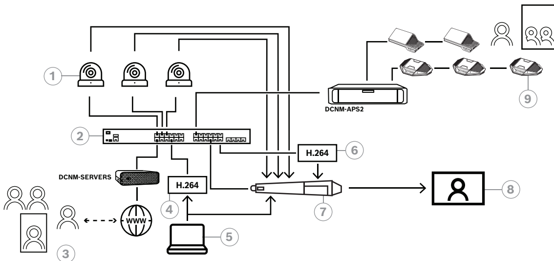
Kuva 8.6: DICENTIS-hybridikokoukset SDI-laitteistokytkennällä
