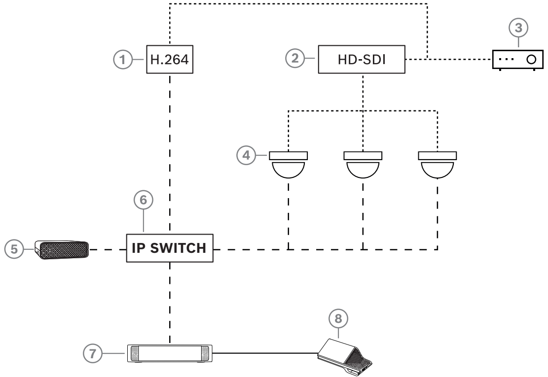
Kuva 3.2: Tyypillinen kamerakoonpano
