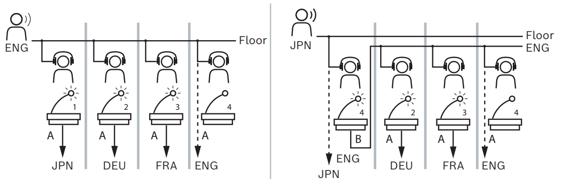
Kuva 5.7: Normaali ja tulkkaus automaattisesta välikielestä
