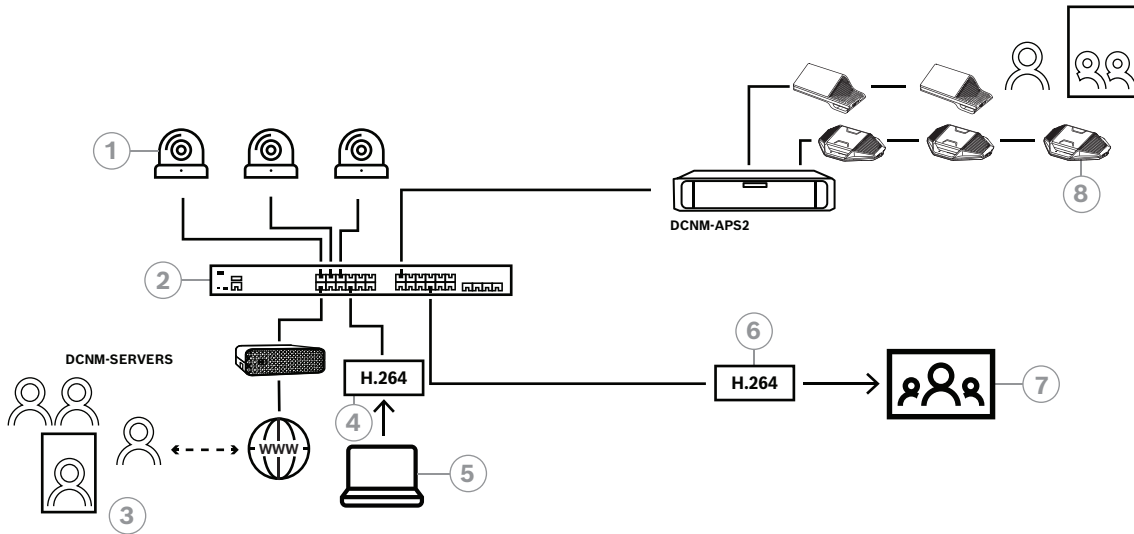
Kuva 8.5: DICENTIS-hybridikokoukset ohjelmistovideokytkennällä
