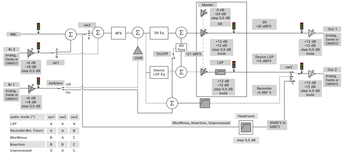
Kuva 5.5: Äänen reititysasetukset
