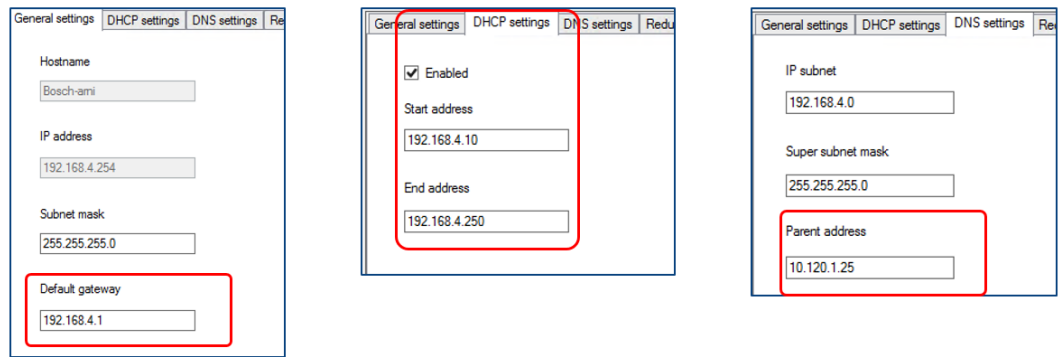
Kuva 5.3: ARNI-järjestelmän määrittys
