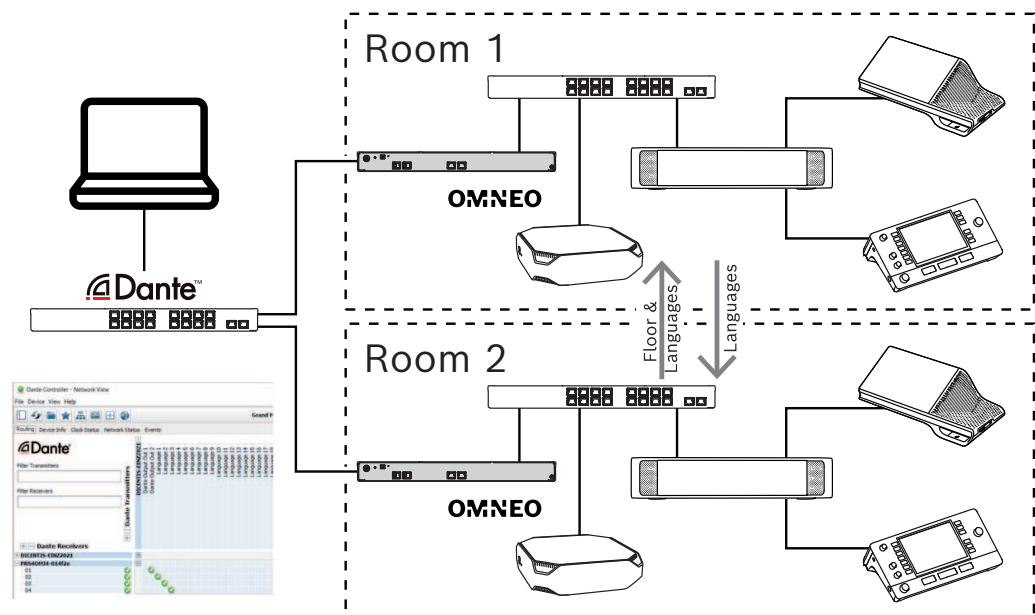
Kuva 5.10: Dante-yhdyskäytävän määrittäminen
