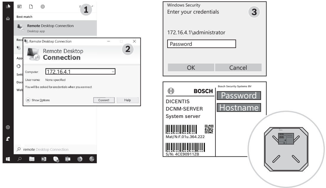
Kuva 14.1: Etätyöpöytäliikennesovellus
