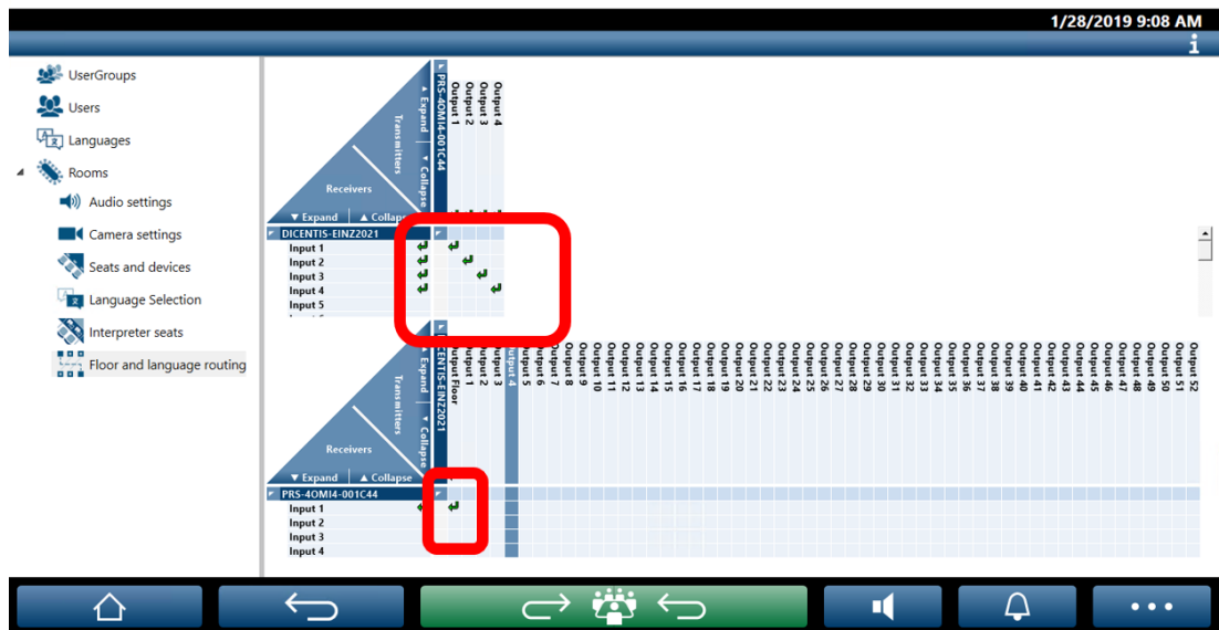
Kuva 5.9: Puhujan ja kielen reititys
