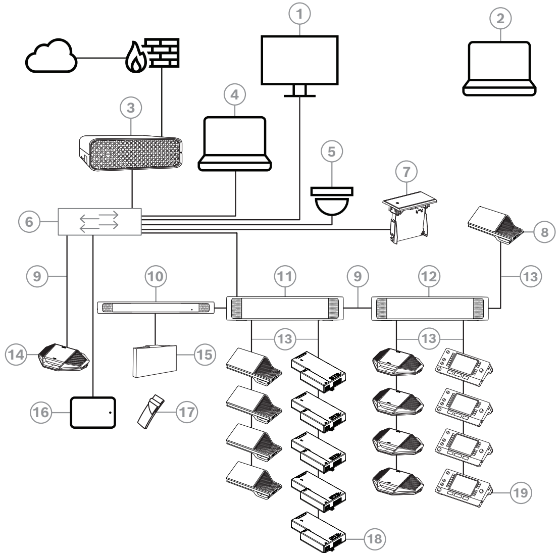
Figura 3.1: Tipica configurazione del sistema per conferenze DICENTIS
