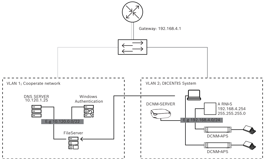
図 5.2: システム図
