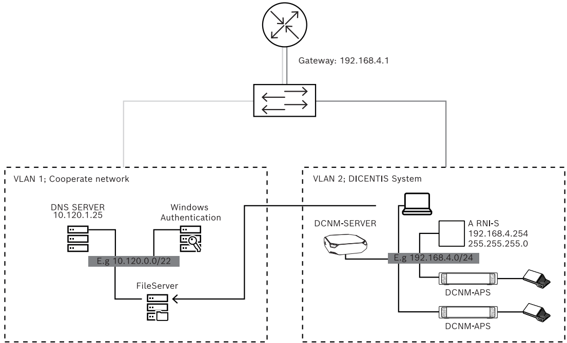
그림 5.2: 시스템 다이어그램
