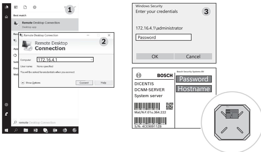
Afbeelding 14.1: Verbinding met extern bureaublad
