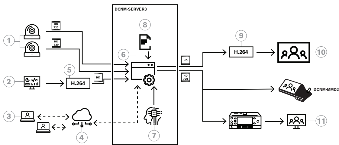
Afbeelding 8.2: Mediagateway - Conceptdiagram
