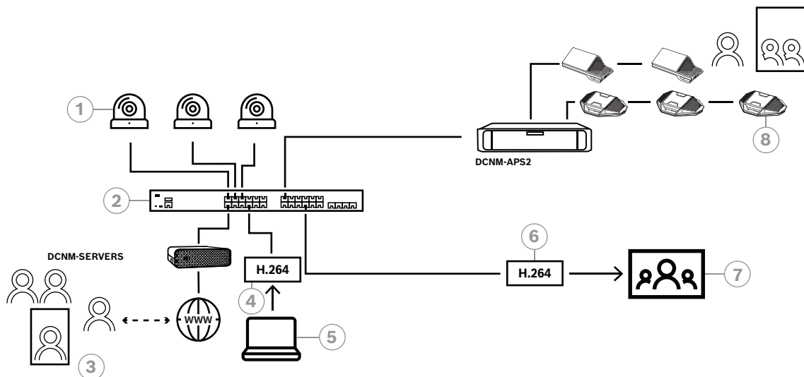
Rysunek 8.5: Hybrydowe spotkania w systemie DICENTIS z użyciem oprogramowania do przetaczania wideo
