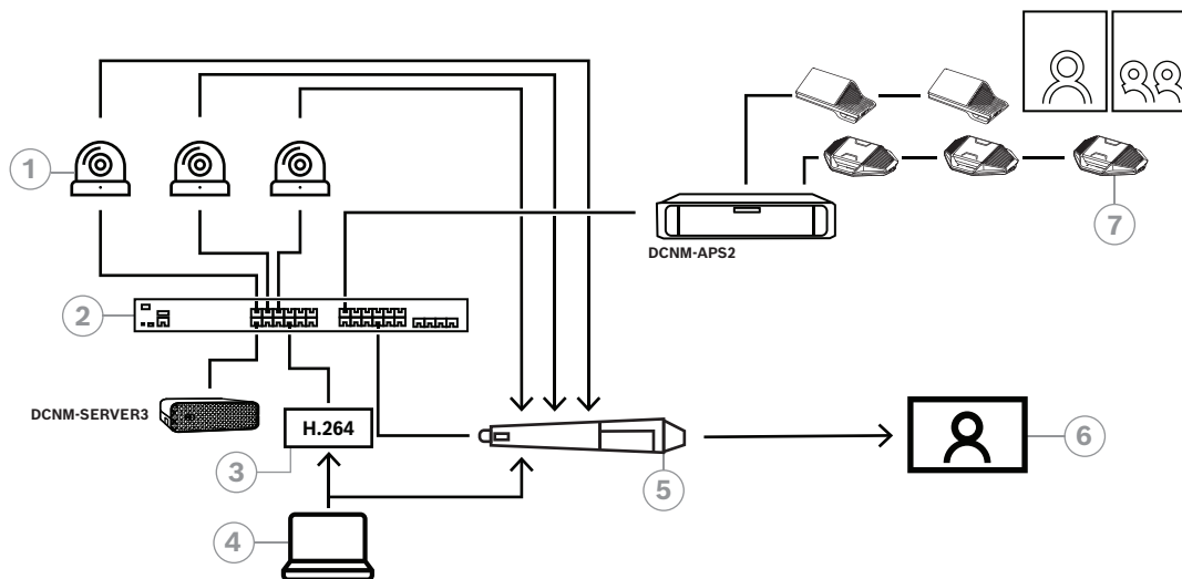
Rysunek 8.4: Samodzielny system DICENTIS z przetwarzaniem sprzętowym SDI
