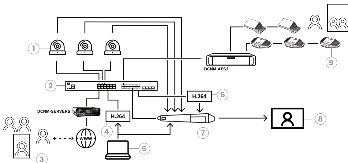
Rysunek 8.6: Hybrydowe spotkania w systemie DICENTIS z użyciem przetłączników sprzętowych SDI
