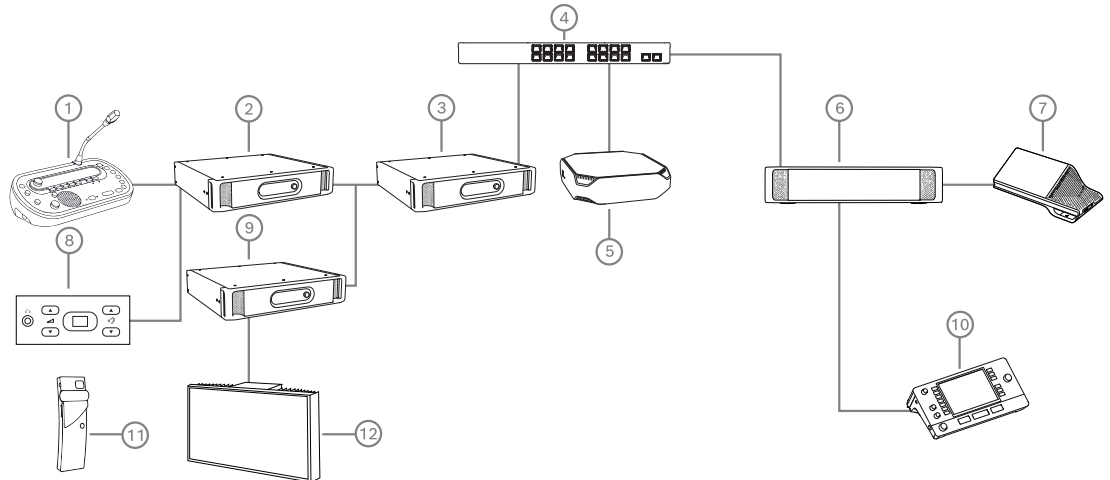
Rysunek 5.8: Współpraca systemów DICENTIS i DCN NG
