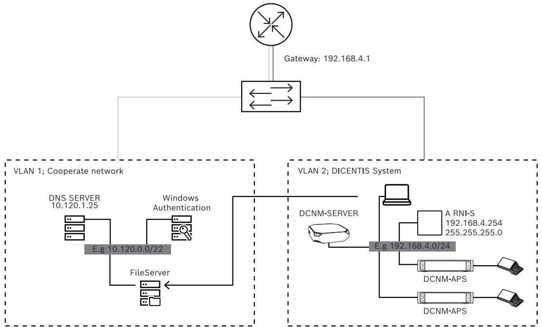
Rysunek 5.2: Schemat systemu
