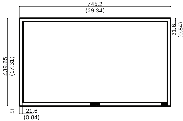
UML-323-90: Vooraanzicht
