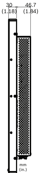
UML-323-90: Zijaanzicht
