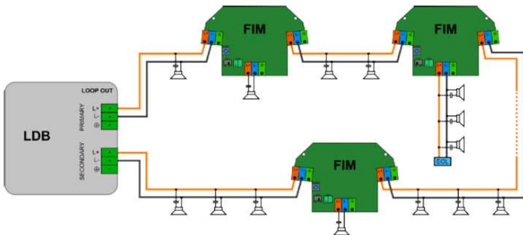
Figura 5.5: Configuración mixta
